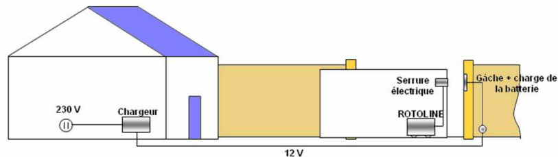
Schéma d'implantation
