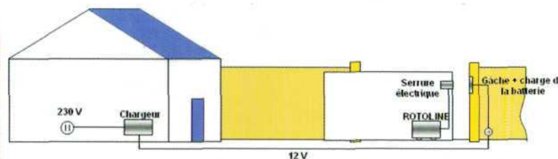
Schéma d'implantation
