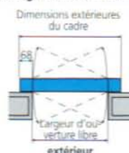
Montage derrière l'embrasure
