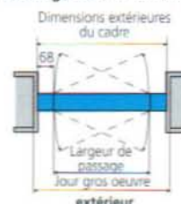
Montage dans l'embrasure
