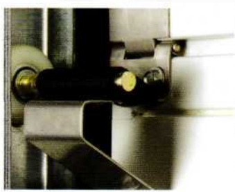
Rouleaux de roulements à billes robustes. Robuste guide di scorrimento a sfera Figure. Ici, pas de protection contre l'écrasement Figura senza sagoma pannello antipizzicamento
