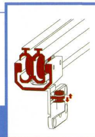
Rail et chariot de roulement en aluminium avec 2 galets à rou- lements à billes (Avec système de réglage en hauteur) Carrello in alluminio e rulli di scorrimento con doppi cuscini a sfera (regolabile in altezza)
