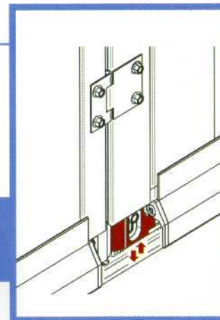
Double brosse d'étanchéité réglable Guarnizione a doppia spazzola, regolabile
