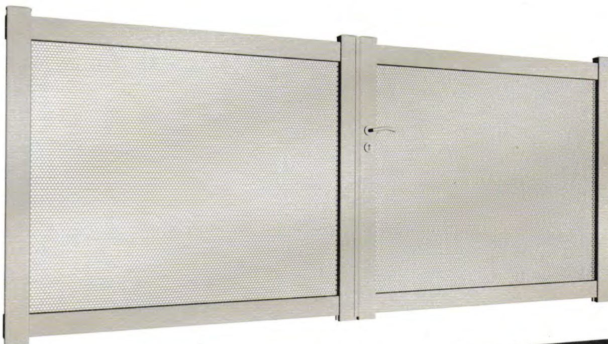
Tucana
