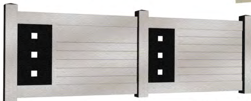
Sagittarius
