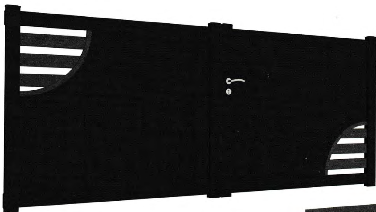
Fidis
