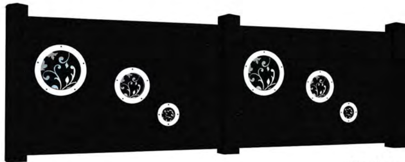
Carina
