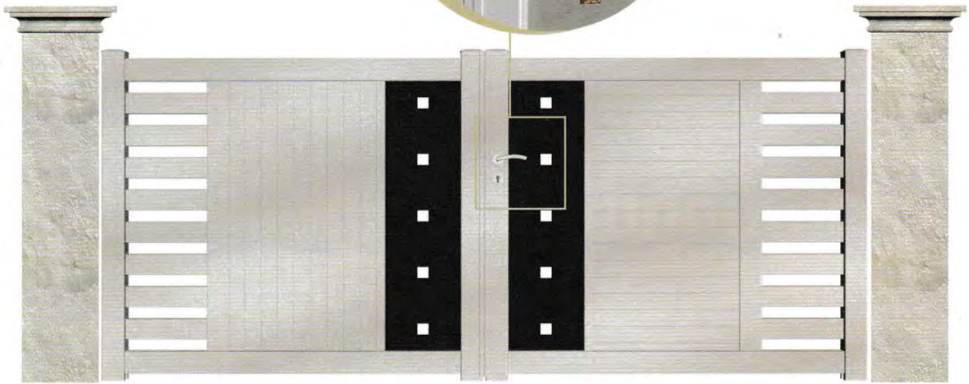
Sagittarius
