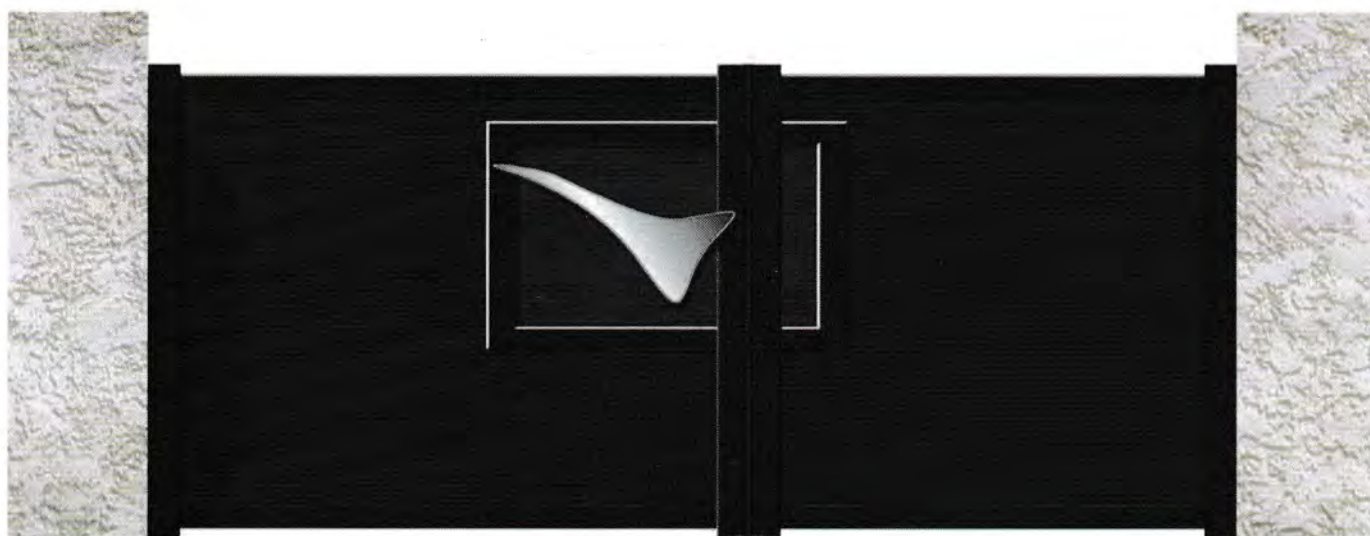
Cetus
