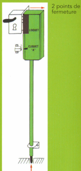
Gâche et tube escamotables
